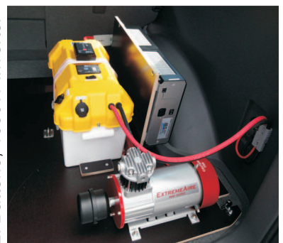
2. Batterie, 1600W Inverter
